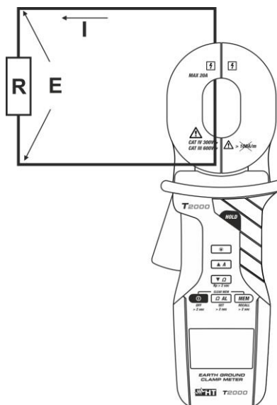
Fig. 6: Mesure de la résistance de la boucle
