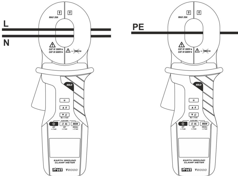
Fig. 23: Misura di corrente di dispersione
