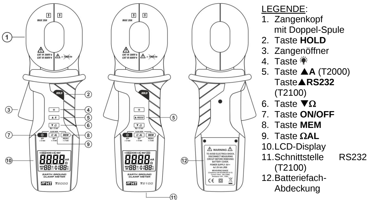
Abb. 1: Beschreibung des Instruments
