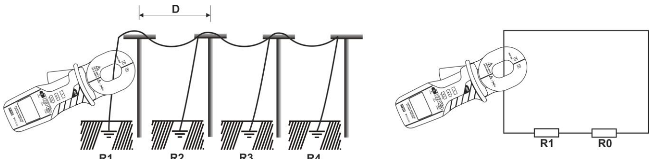
Fig. 9: Collegamento dello strumento ad un sistema multi-dispersori
