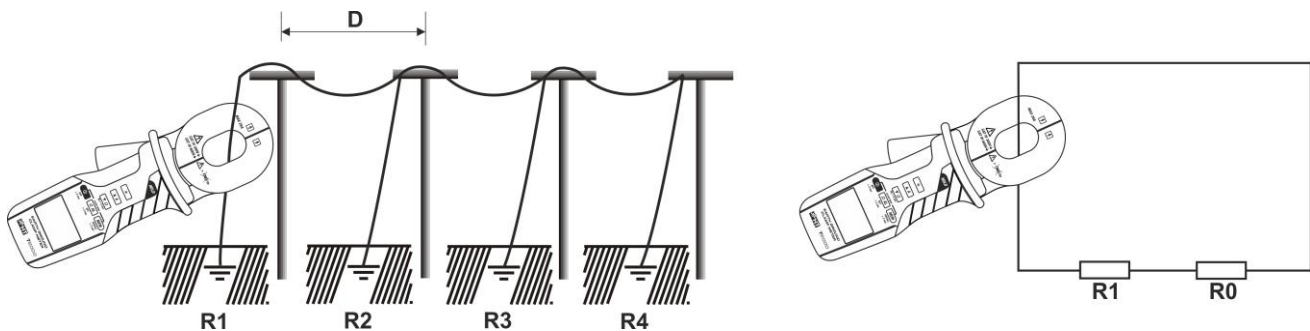
Fig. 9: Ligação do instrumento num sistema multi-dispersores
