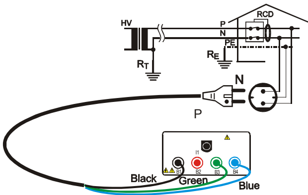
Instrumentenverbindung für 230V Ein-Phasen RCD Prüfung
