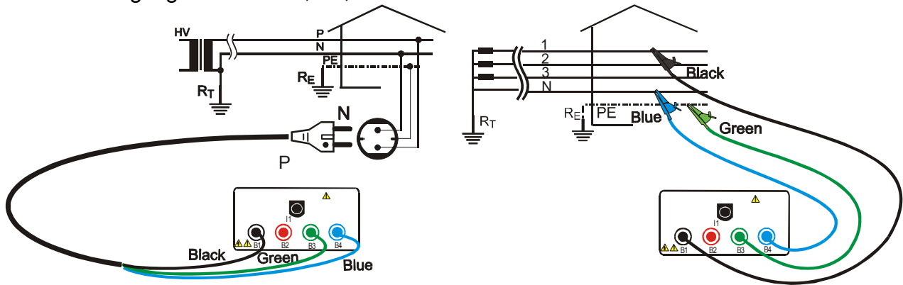
Instrumenten- Beschaltung für P-PE Test in einem 400V Drei-Phasen System
