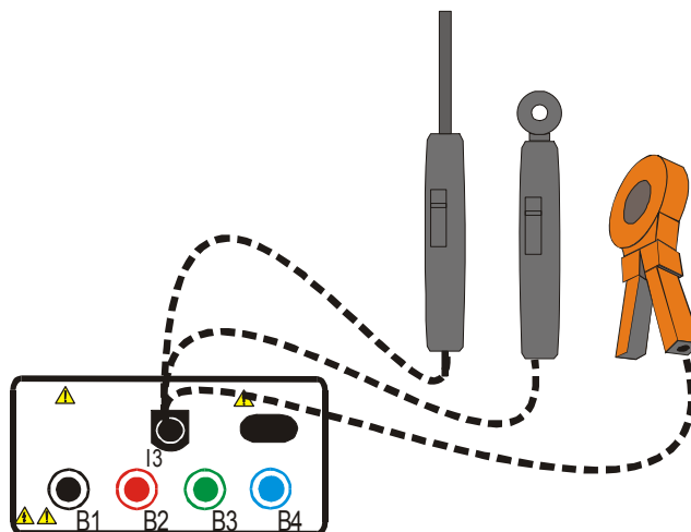
Beispiel für Verbindungen mit externen Prüfsonden
