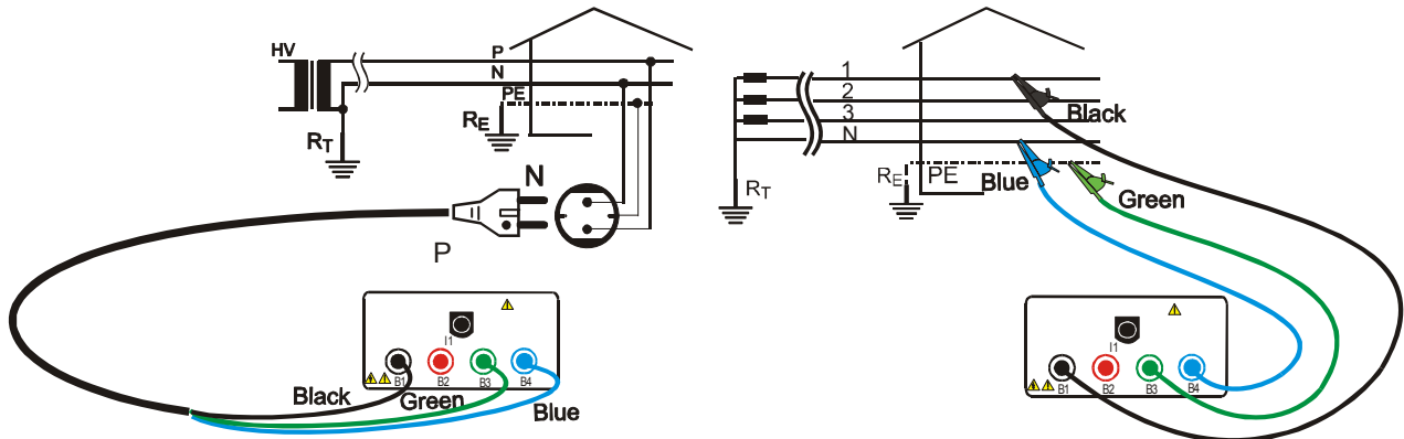
Instrumenten- Beschaltung für P-N Test in einem 400V Drei-Phasen System
