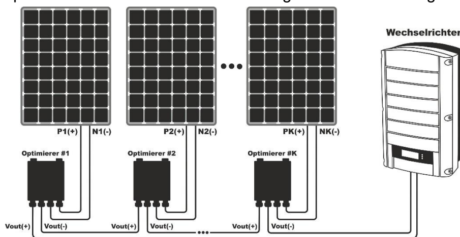
Abb. 20: Verbindung eines PV-Strings mit Leistungsoptimierern
