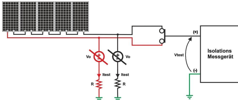
Abb. 19: Schema und Ersatzschaltung von Methode 2
