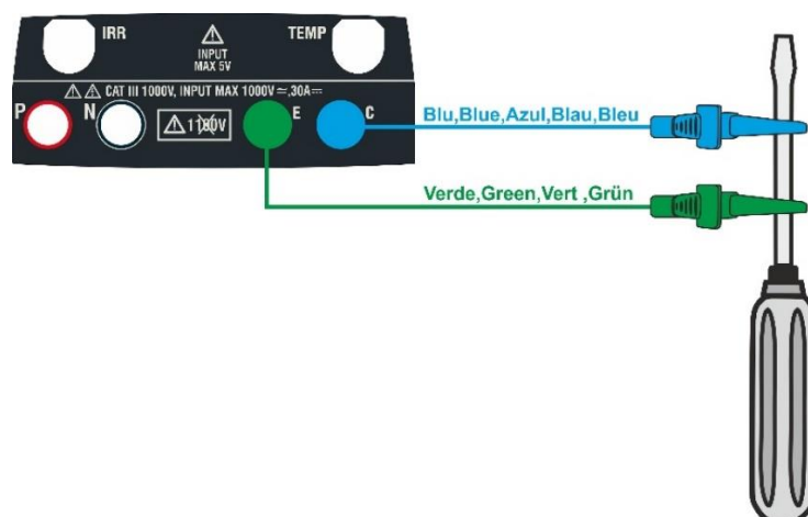
Abb. 5: Kompensation des Widerstands der Messkabel
