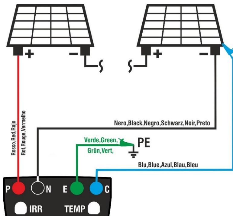
Abb. 11: Verbindung für IVCK-Tests ohne Fernstation und ohne Bestrahlungsstärkemessung
