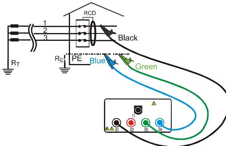
Instrumenten- Beschaltung für den P-PE Test in einem 400V Drei-Phasen-System ohne Neutraleiter
