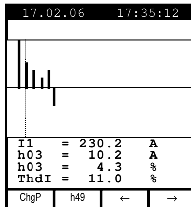
Beispiel - Bildschirm für 3 Phasen-Modus
