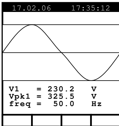
Beispiel - Bildschirm für Ein-Phasen-System
