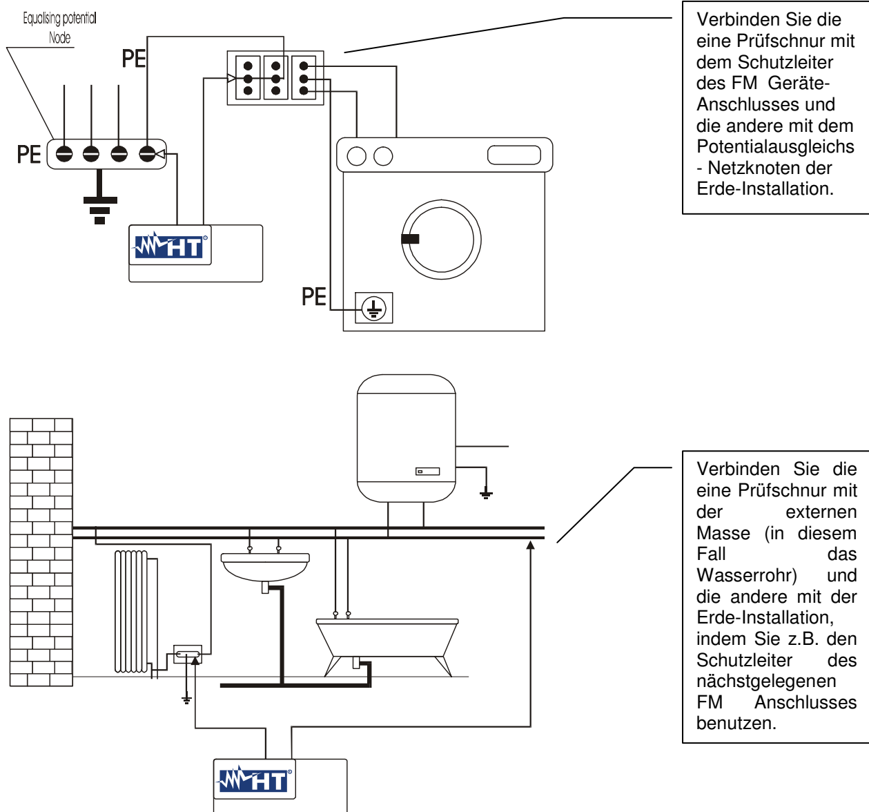
Beispiele für eine Durchgangsmessung an Leitungen
