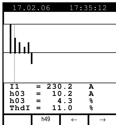
Beispiel des Schirms im Einphasenmodus
